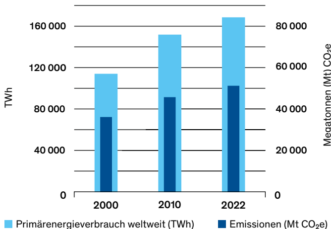
Der weltweite Primärenergiebedarf und daraus resultierende CO 2 e-Emissionen
