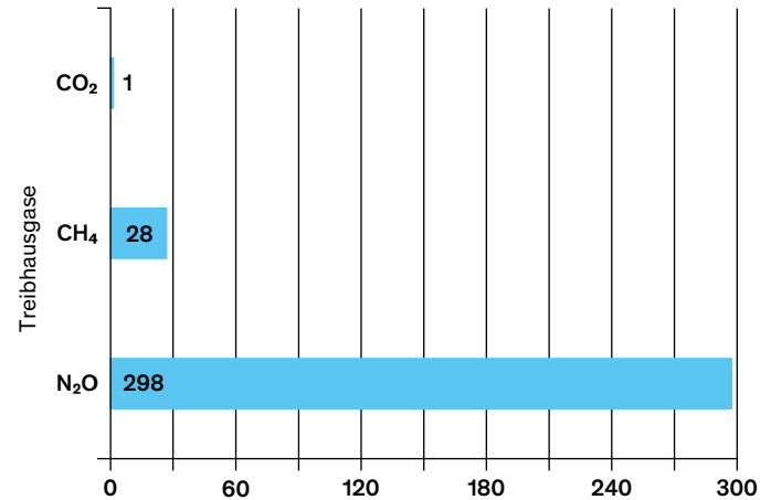
Erwärmungspotenzial im Vergleich
