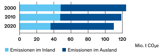
Treibhausgasemissionen, die mit der Schweizer Endnachfrage nach Gütern und Dienstleistungen entlang der Wertschöpfungskette verbunden sind
