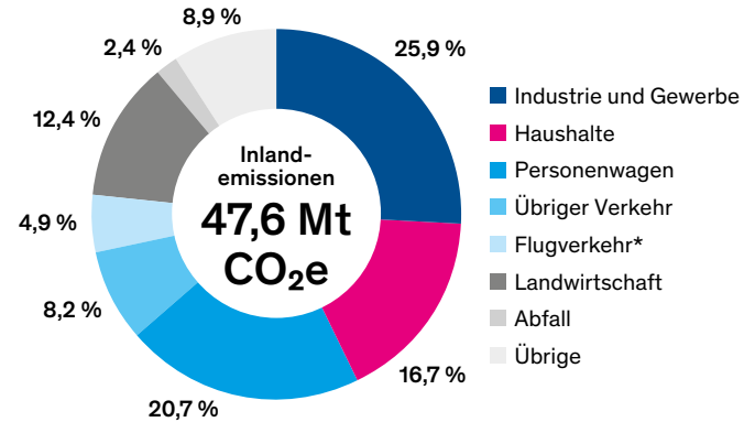
Treibhausgasemissionen in der Schweiz, unterteilt nach einzelnen Sektoren (2021) inklusive Flugverkehr
