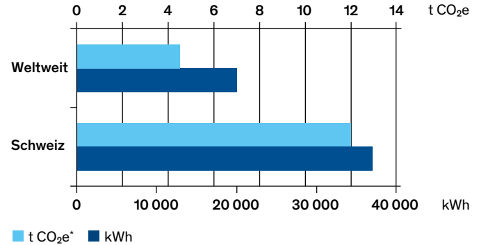
Vergleich des globalen Energieverbrauchs und der Treibhausgasemissionen pro Kopf weltweit (2022) und in der Schweiz (2021)
