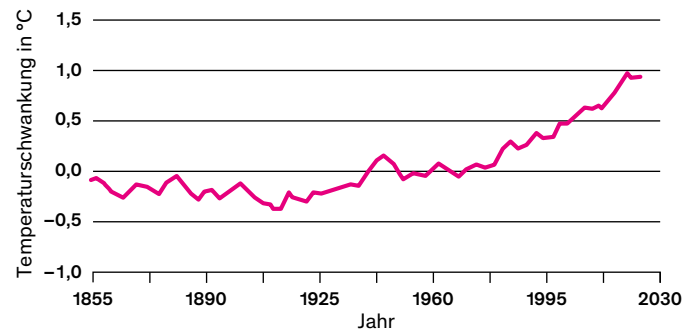
Temperaturentwicklung, global, seit der Industrialisierung
