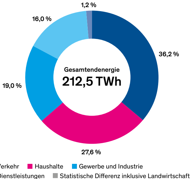
Endenergieverbrauch in der Schweiz nach Sektoren (2022)
