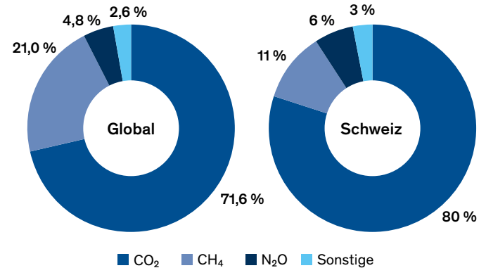
Die Zusammensetzung der Treibhausgasemissionen – global und in der Schweiz
