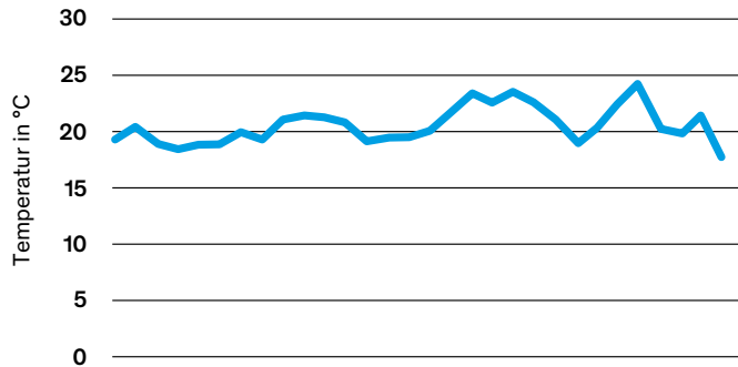
Die Lufttemperatur (Tagesmitte) im Juni 2023 in Zürich-Fluntern
